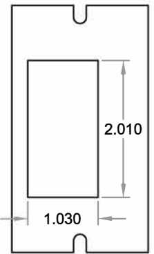
DP009 For Ortronics 2/TJ Bezel
